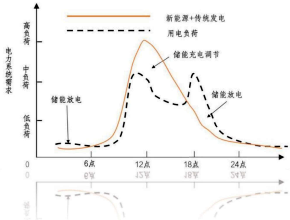
图表：电源侧，储能吸收过剩电力，减少弃电、增加并网
